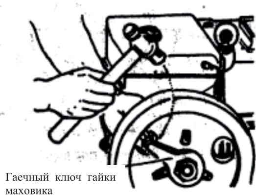
Рис. 25 Ослабление гайки маховика
